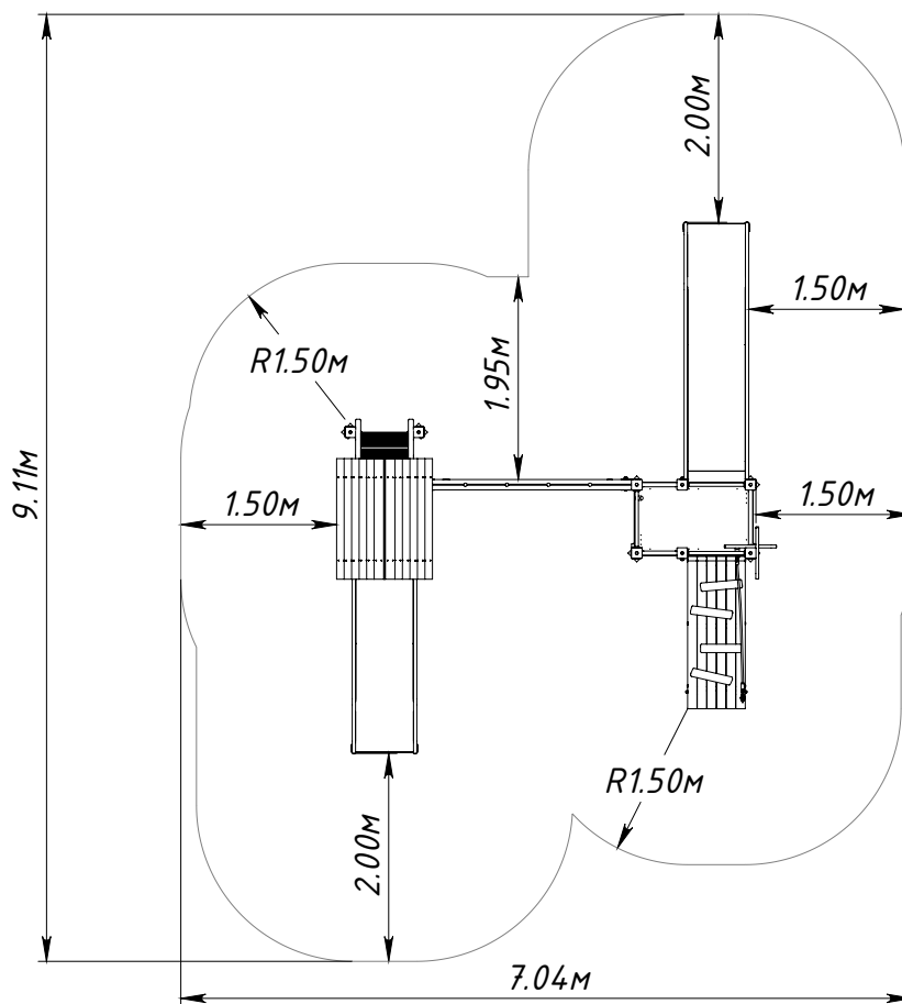
Рисунок 2 — Граница зоны приземления
