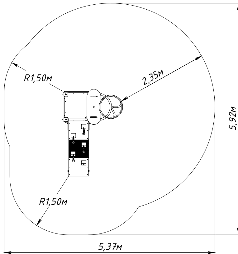
Рисунок 1 — Основные габаритные размеры
